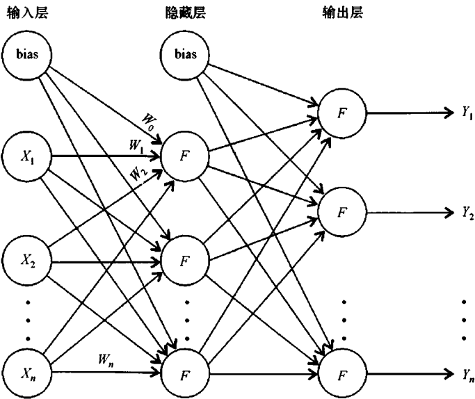
图 1 多层感知器神经网络结构示意图
