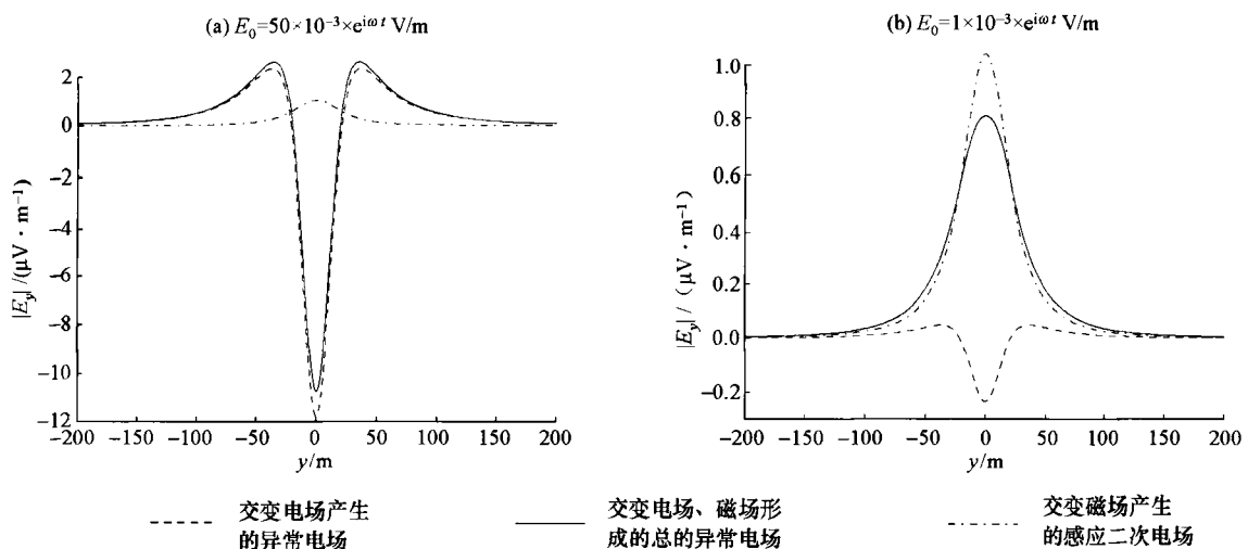
图 5 地表主剖面沿 y 轴方向异常电场强度 E_y 曲线
