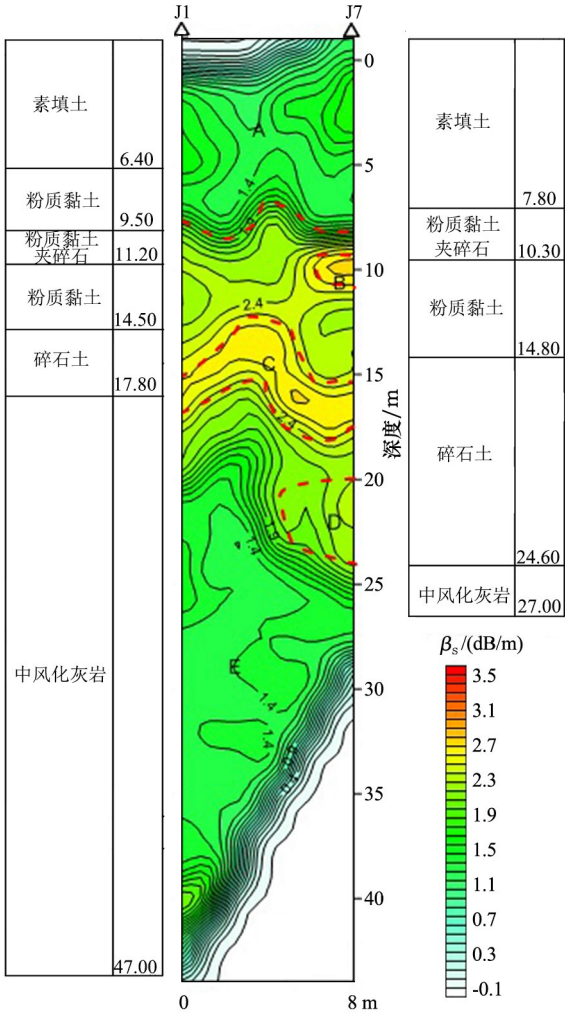
图 3 检测孔 J1-J7 电磁波间跨孔检测成果
