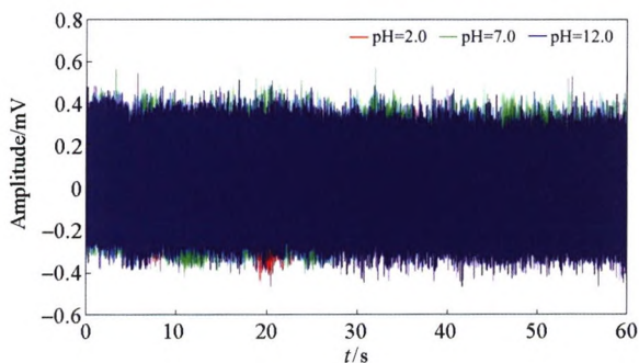
图 3 石墨电极在不同 pH 下的极差 (20℃)
