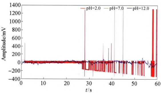
图 1 Cu-CuSO 4 电极在不同 pH 下的极差 (20℃)
