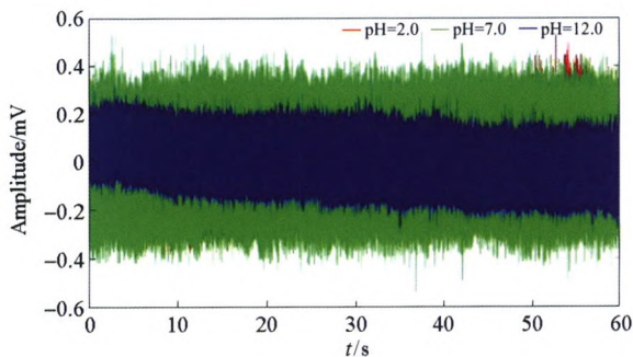
图 6 石墨电极在不同 pH 下的极差 (90℃)
