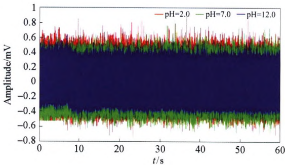
图 2 铅电极在不同 pH 下的极差 (20℃)
