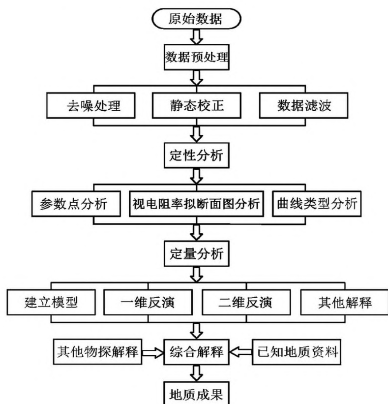
图1 广域电磁法数据处理流程
