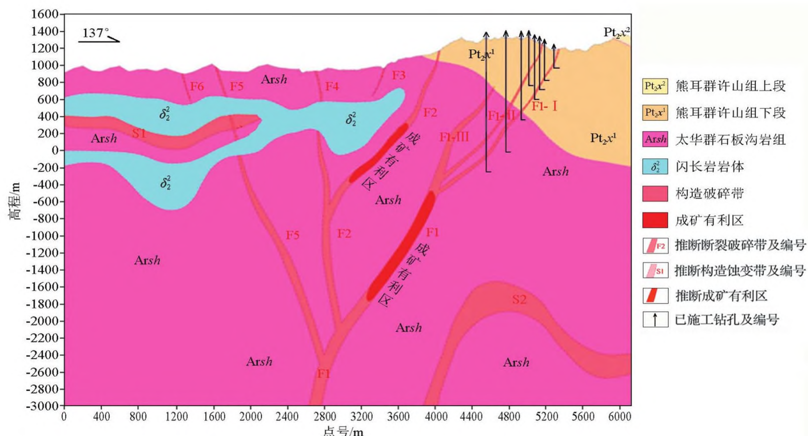
图 3 GY01 线解释成果剖面
