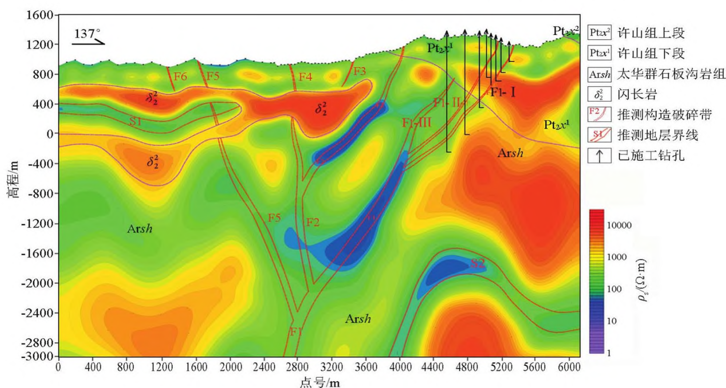
图2 GY01线广域电磁法二维反演电阻率断面及综合解释成果
