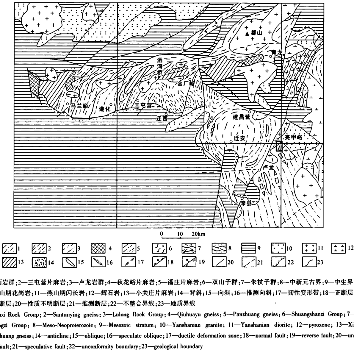
图 1 冀东太古宙杂岩地质构造略图 [4]
