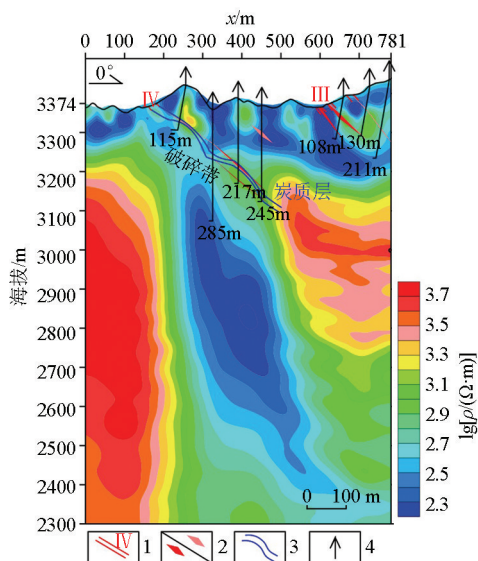
图 7 打柴沟 8 勘探线地质—WFEM 反演成果
