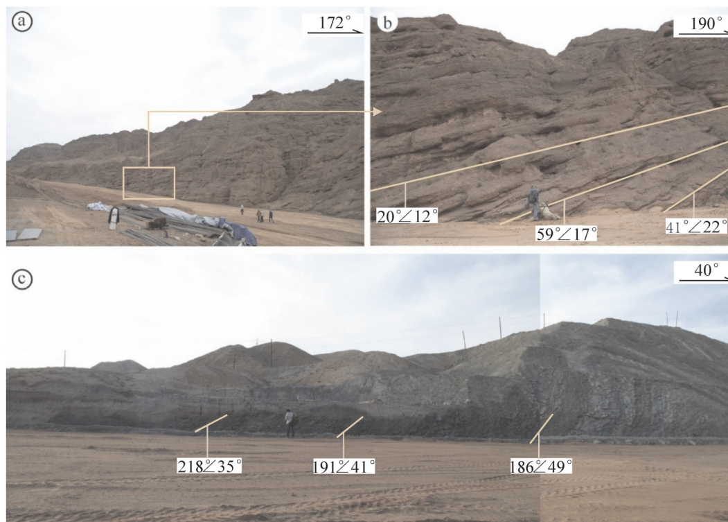
图5 平山湖盆地内发育的生长地层 (a, b—仁宗口背斜北翼生长地层; c—平易背斜南翼生长地层)
