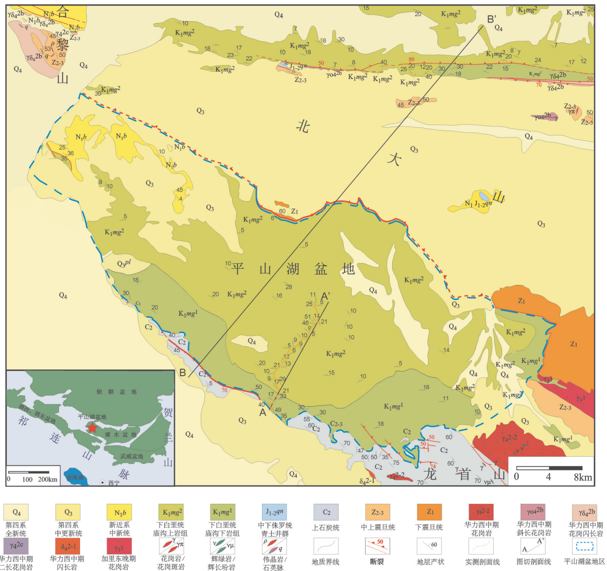
图1 平山湖盆地地质图
