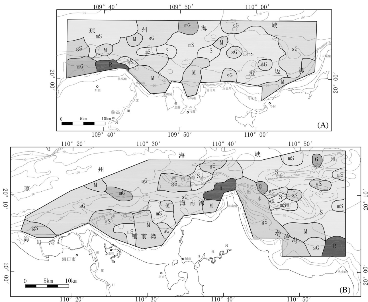
图2 研究区底质类型图(A—西区;B—东区)
