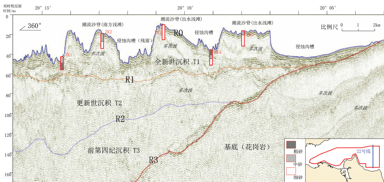
图5 研究区22号线综合地震剖面图
