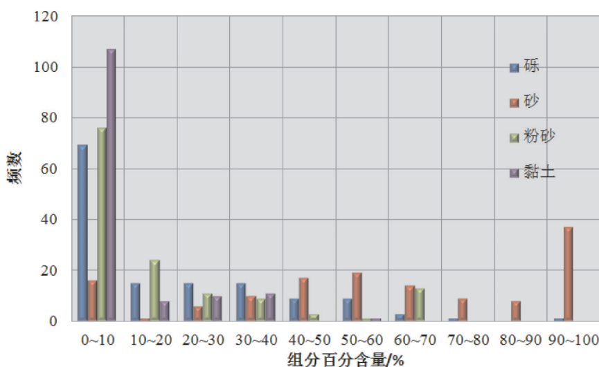
图3 沉积物粒度组分统计
