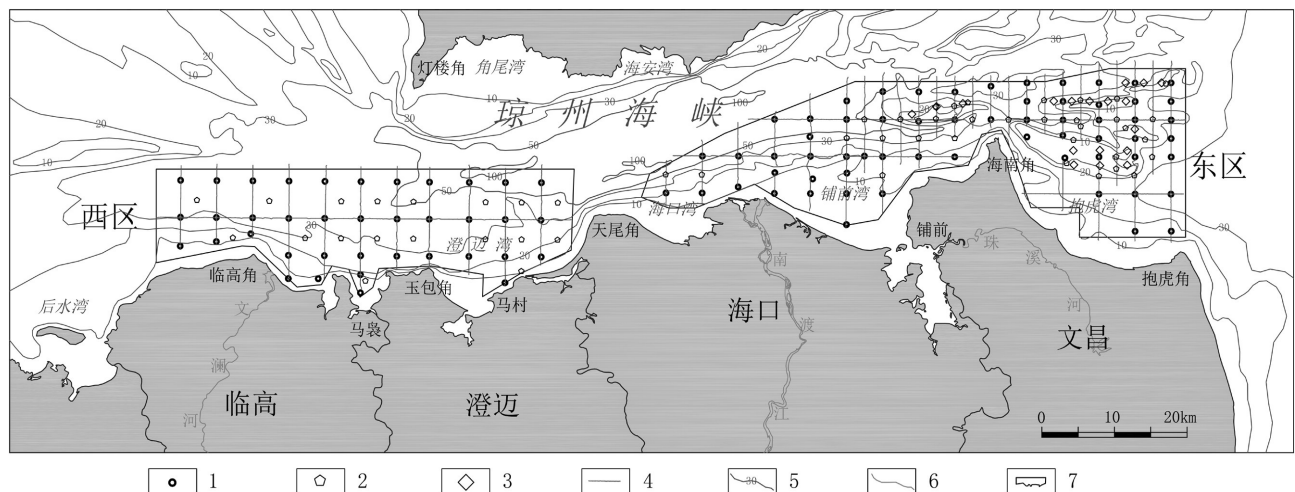
图1 研究区范围及采样位置图
