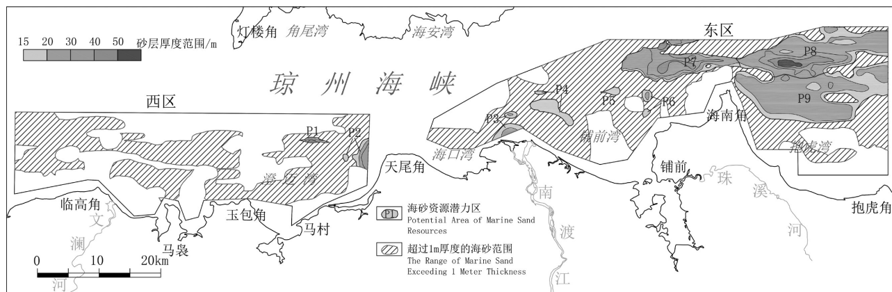
图7 研究区海砂资源潜力图
