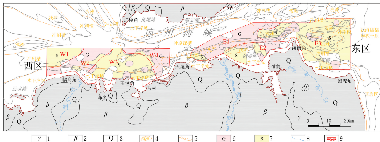
图4 研究区海砂分布图
