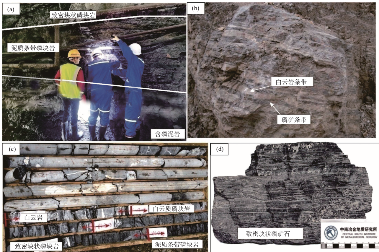
图4 磷矿石野外地质特征
