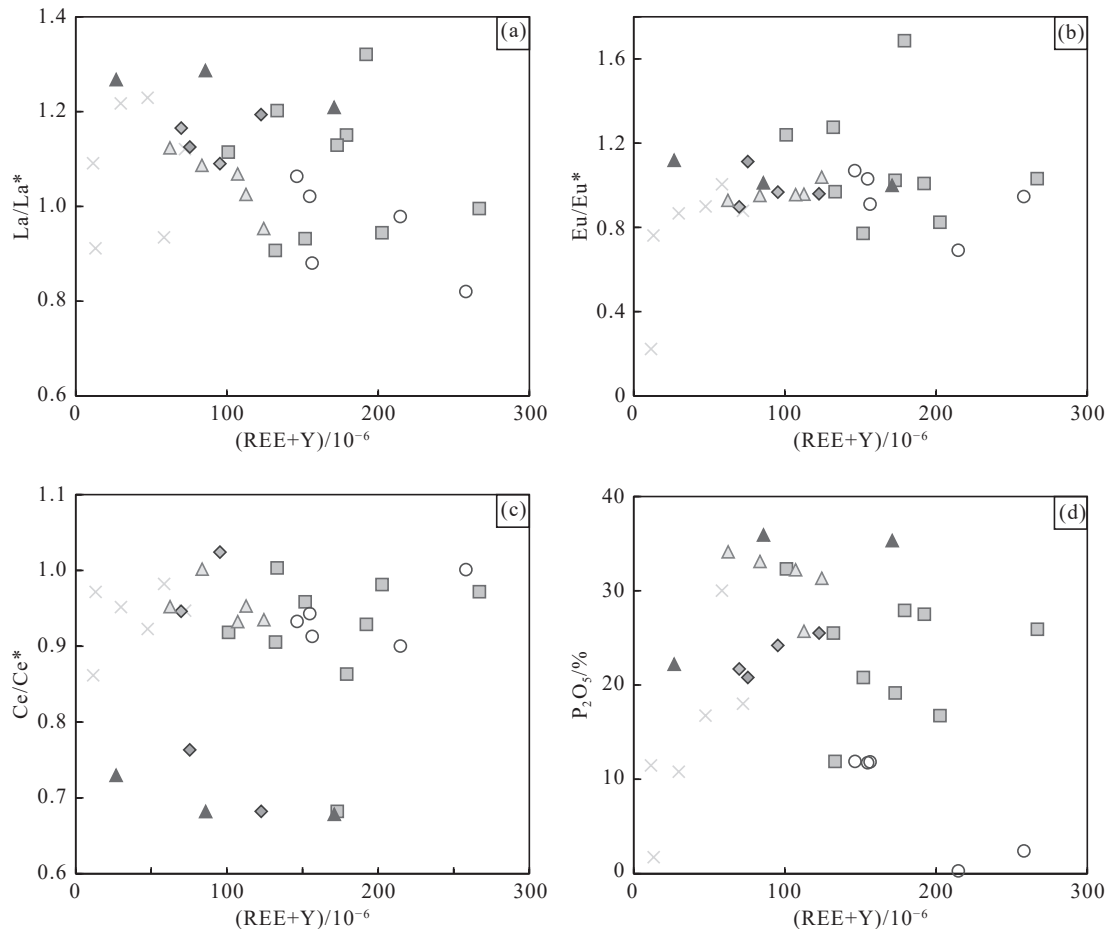
图 9 磷块岩稀土元素含量图解(图例同图 8)
