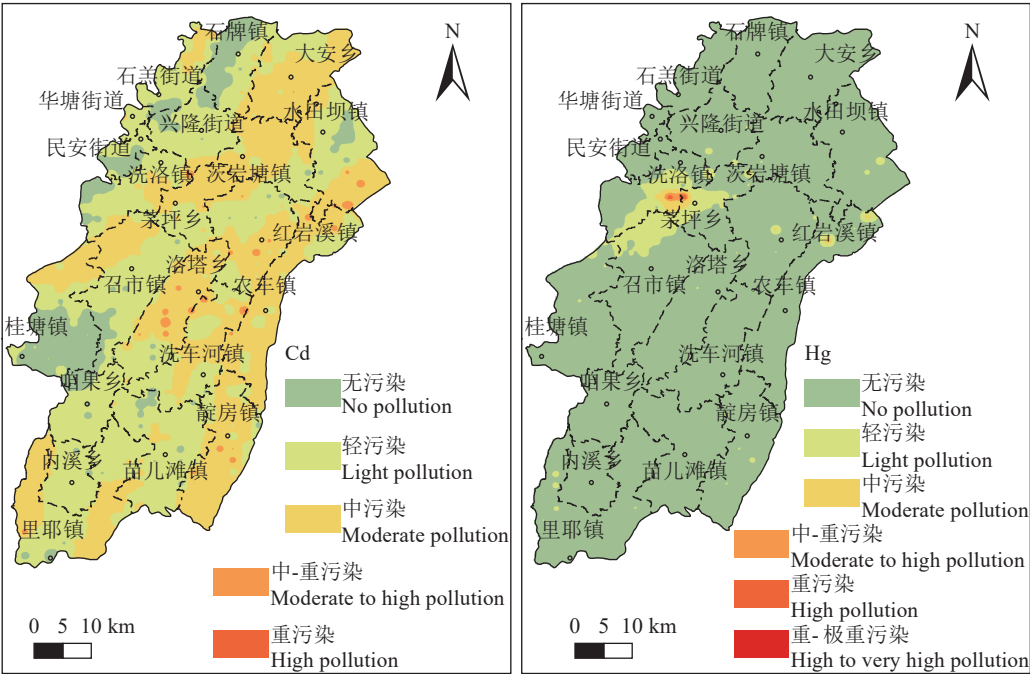
图 3 土壤 Cd 与 Hg 的污染等级分布 Fig.3 Distribution of pollution levels of Cd and Hg in soil
