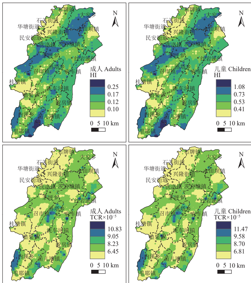
图 8 HI 与 TCR 空间分布格局 Fig.8 Spatial distribution patterns of HI and TCR
