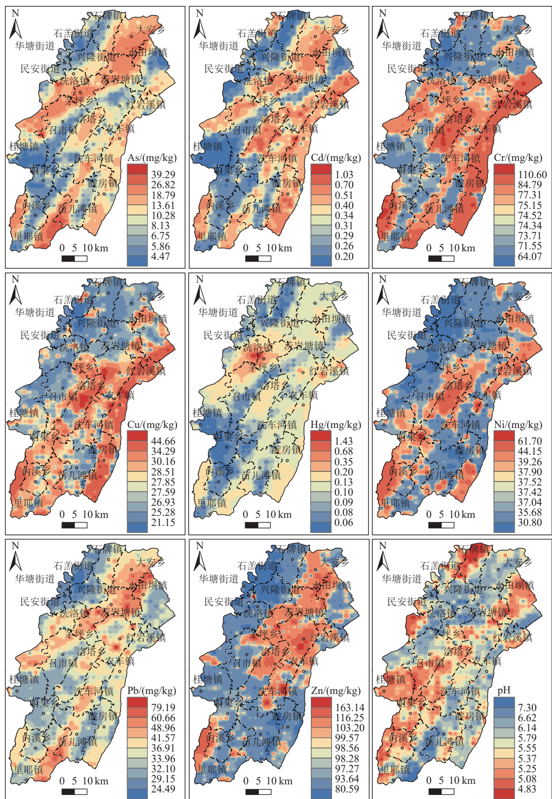
图 2 龙山县土壤重金属含量空间分布图
