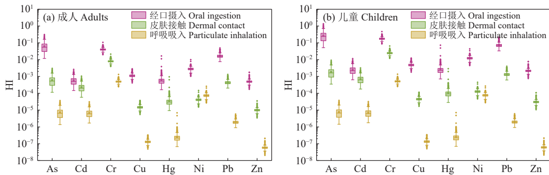
图 4 不同重金属和暴露途径的非致癌风险指数
