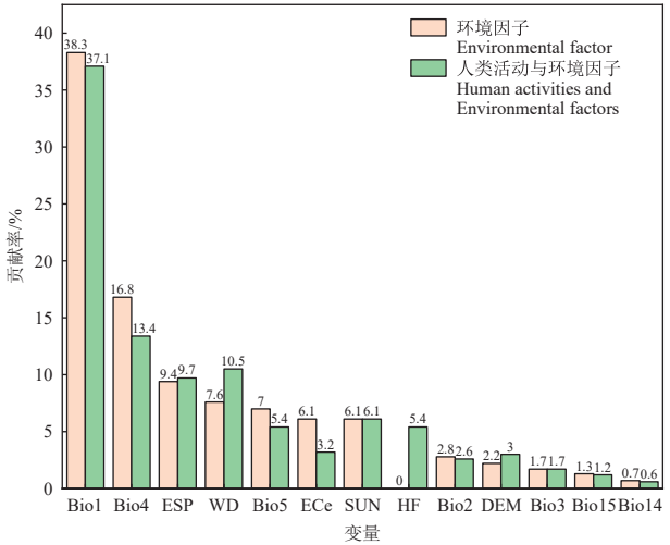
图 2 MaxEnt 模型中变量的贡献度 Fig.2 Contribution of variables in the MaxEnt model
