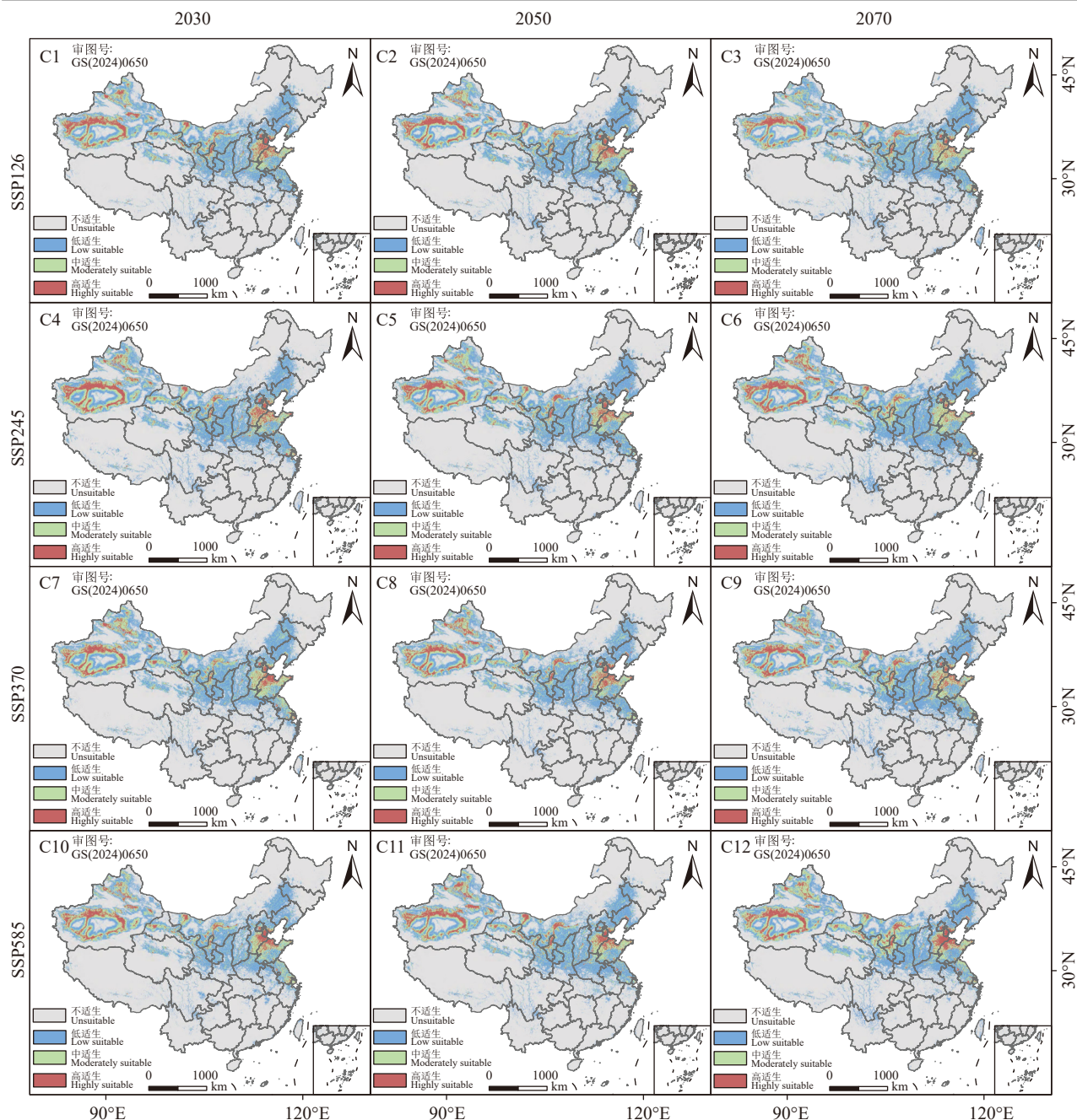
图4 未来不同气候情景下柽柳的潜在适生区
