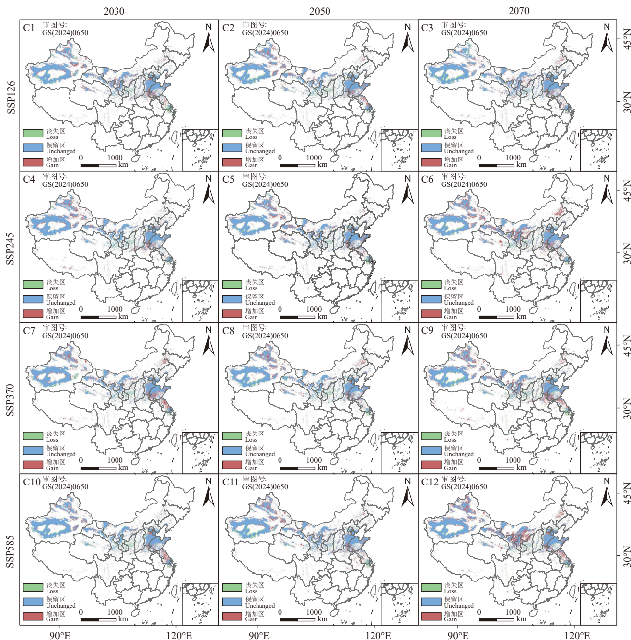
图6 不同气候情境下怪柳适生区空间变换格局
