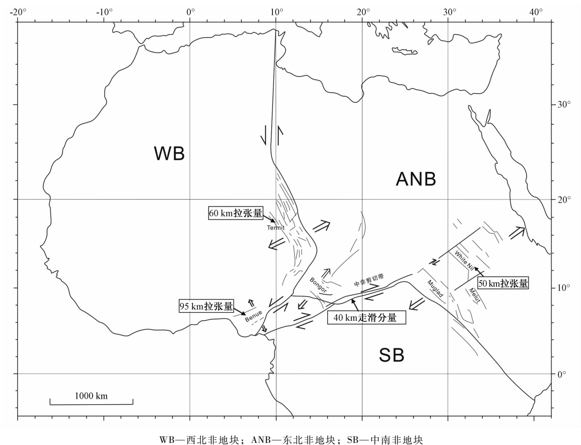
图 5 非洲裂谷系白垩纪伸展量或滑移量图 [14]
