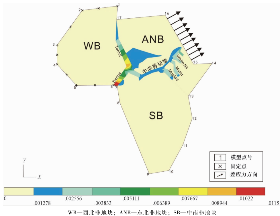
图 4 早白垩世非洲大陆的张应变等值线图
