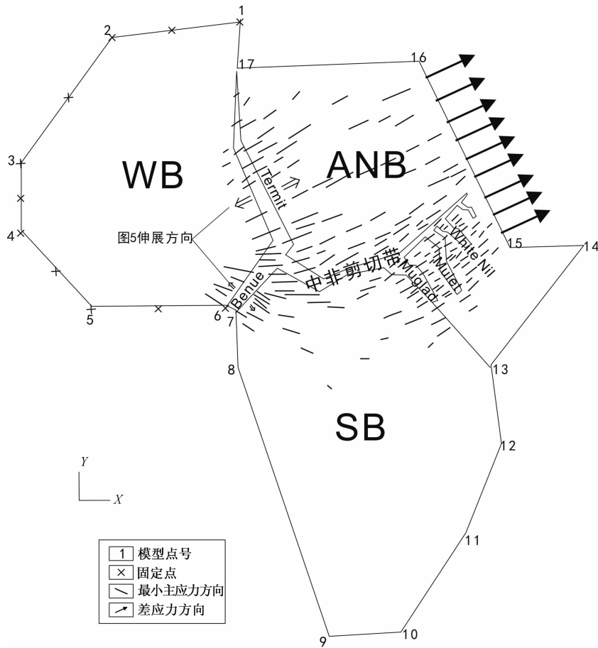
图 6 早白垩世非洲大陆的最小主压应力方向图
