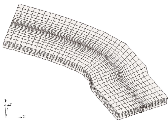
图2 有限元模型及网格划分
