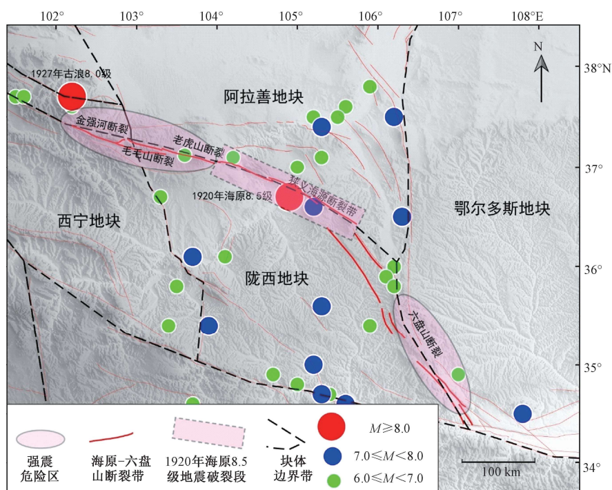
图 1 研究区构造特征及历史强震
