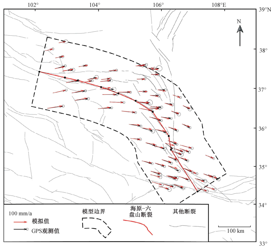
图 5 模拟速度场和 GPS 观测结果的对比
