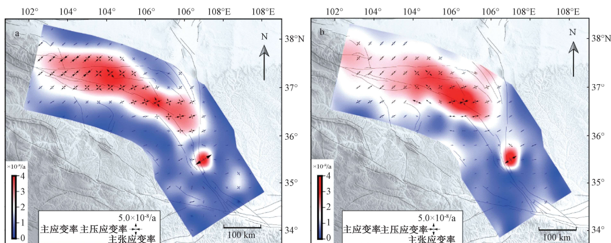
图中色卡对应颜色表示最大剪应变率大小, 十字叉表示主压、主张应变率大小和方向
