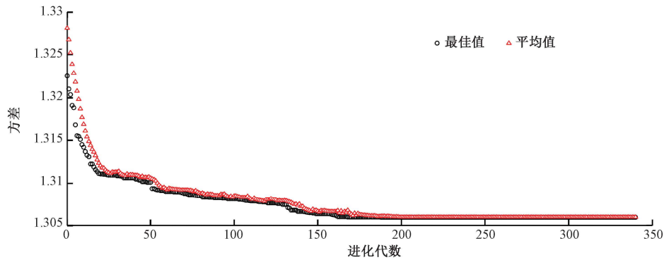
图 4 目标函数收敛过程
