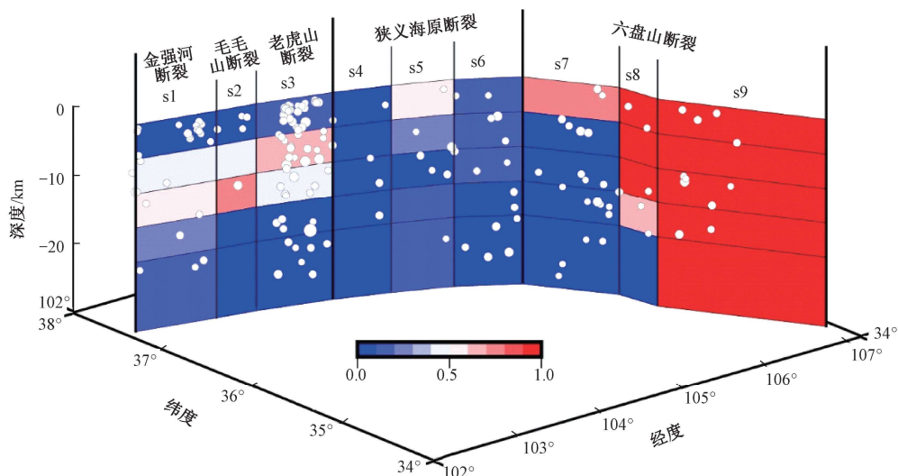
色块代表每个分块平行断层面的剪切模量和周围介质剪切模量的比值,白色圆圈代表距断层两侧各10 km范围内小震(3.0级以上)精定位结果在断层面的投影
