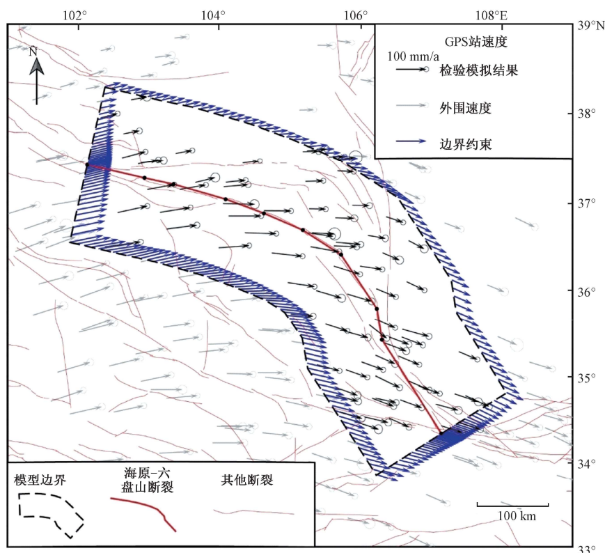
图3 研究区 GPS 观测速度场 (1999—2016 年)
