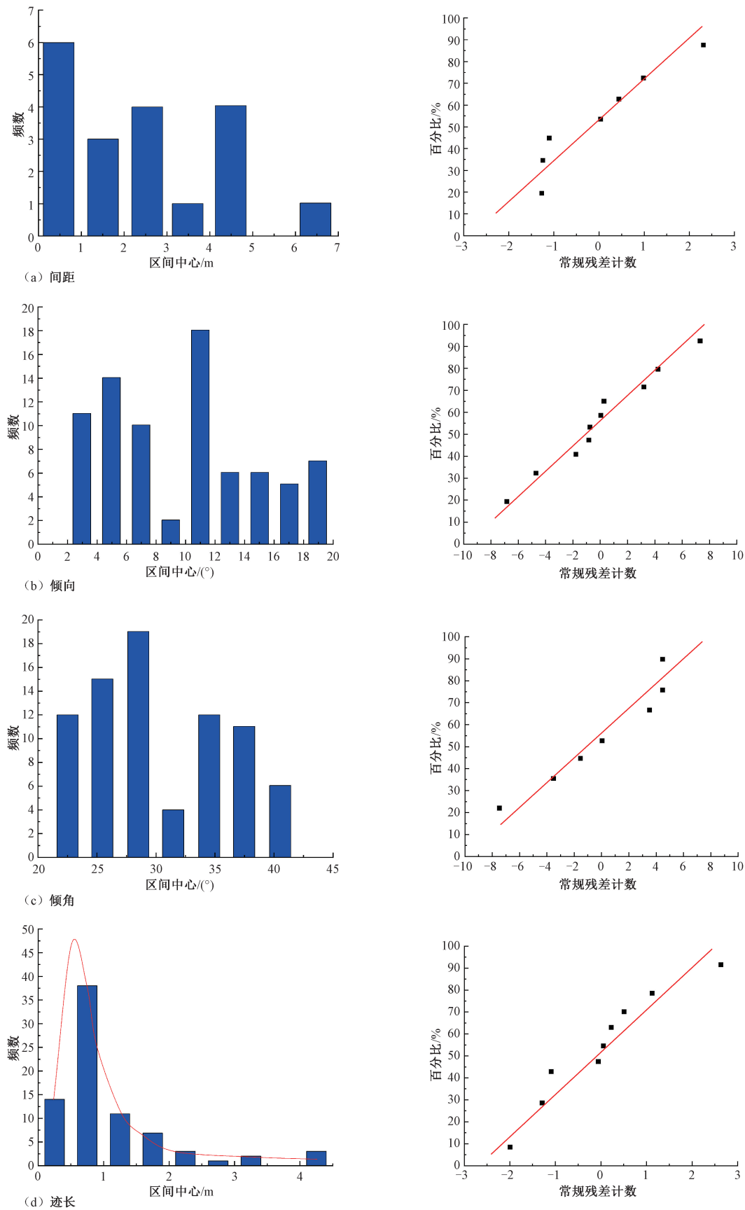
图 3 平洞 PD02 第①组缓倾角结构面概率分布及残差图
