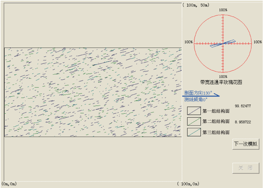
图 4 PD02 缓倾角结构面网络模拟结果
