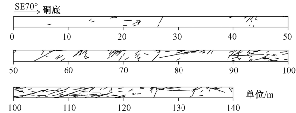
图 5 PD02 缓倾角结构面展布图
