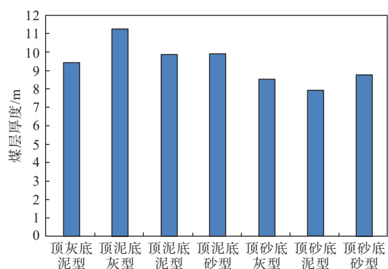
图5 不同顶底板岩性组合的煤层厚度统计直方图
