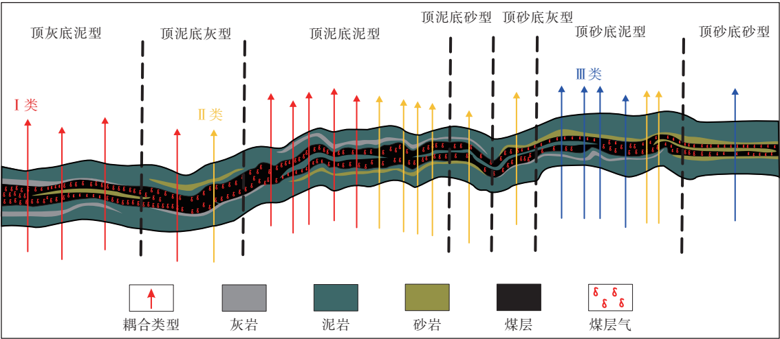
图 13 深层煤层气的富集耦合模式 Fig. 13 Coupling model of deep coalbed methane enrichment
