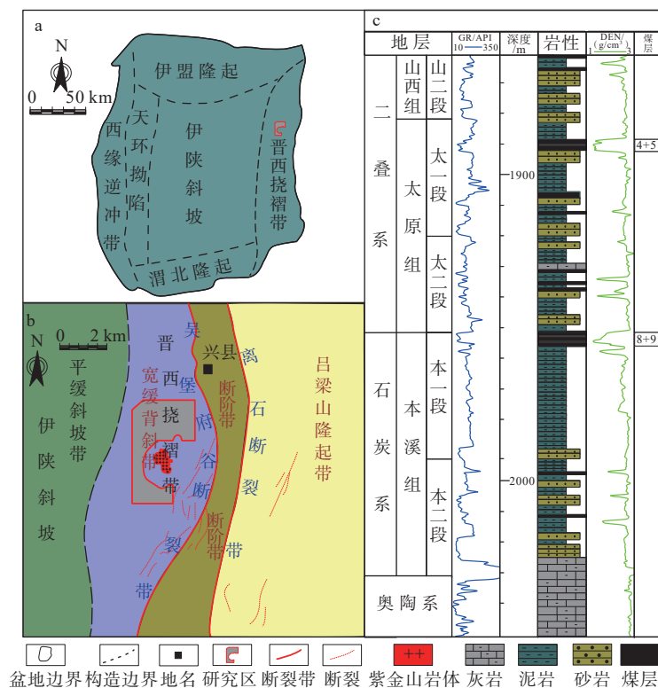
图 1 研究区构造位置图及地层柱状图
