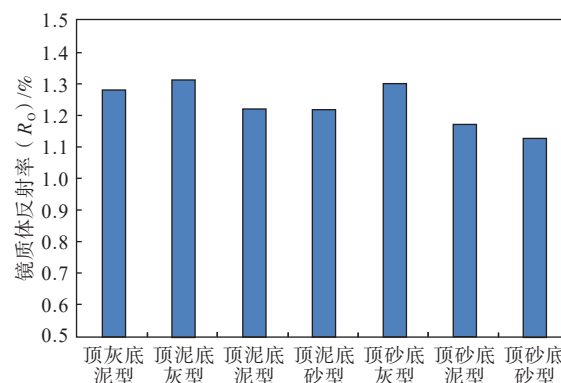
图6 不同顶底板岩性组合的煤层镜质组反射率直方图
