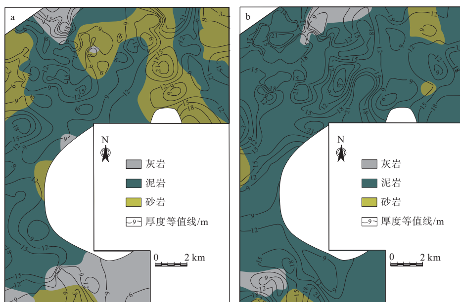
图4 临兴地区深层煤层顶底板厚度等值线图
