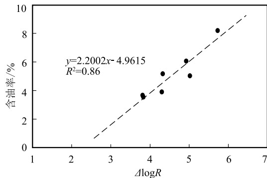
图11 三塘湖盆地油页岩 \Delta\log R 与含油率关系图解
