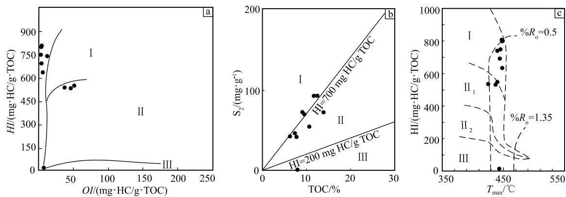
图 4 三塘湖盆地芦草沟组油页岩有机质类型及成熟度
