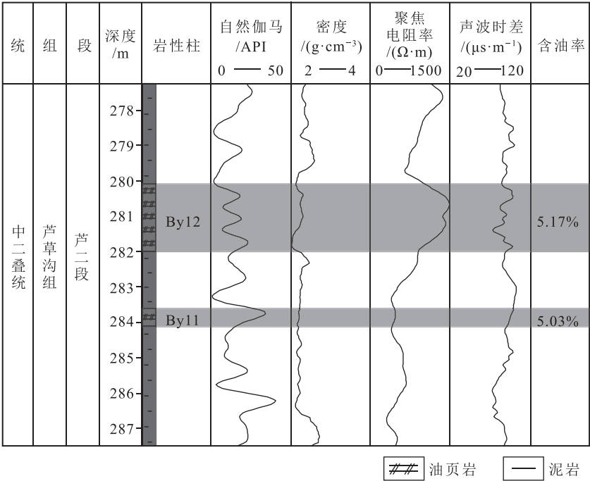
图 5 三塘湖盆地巴油页 1 井 By12 油页岩测井响应特征
