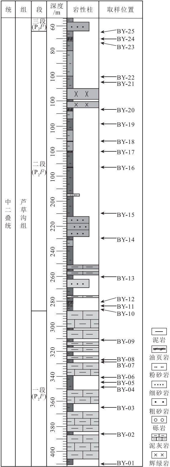
图 3 巴油页 1 井取样位置图 Fig. 3 Sampling point of borehole Byy-1
