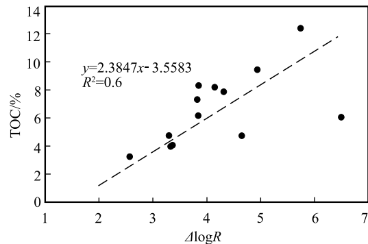
图 8 \Delta \log R 与 TOC 相关性
