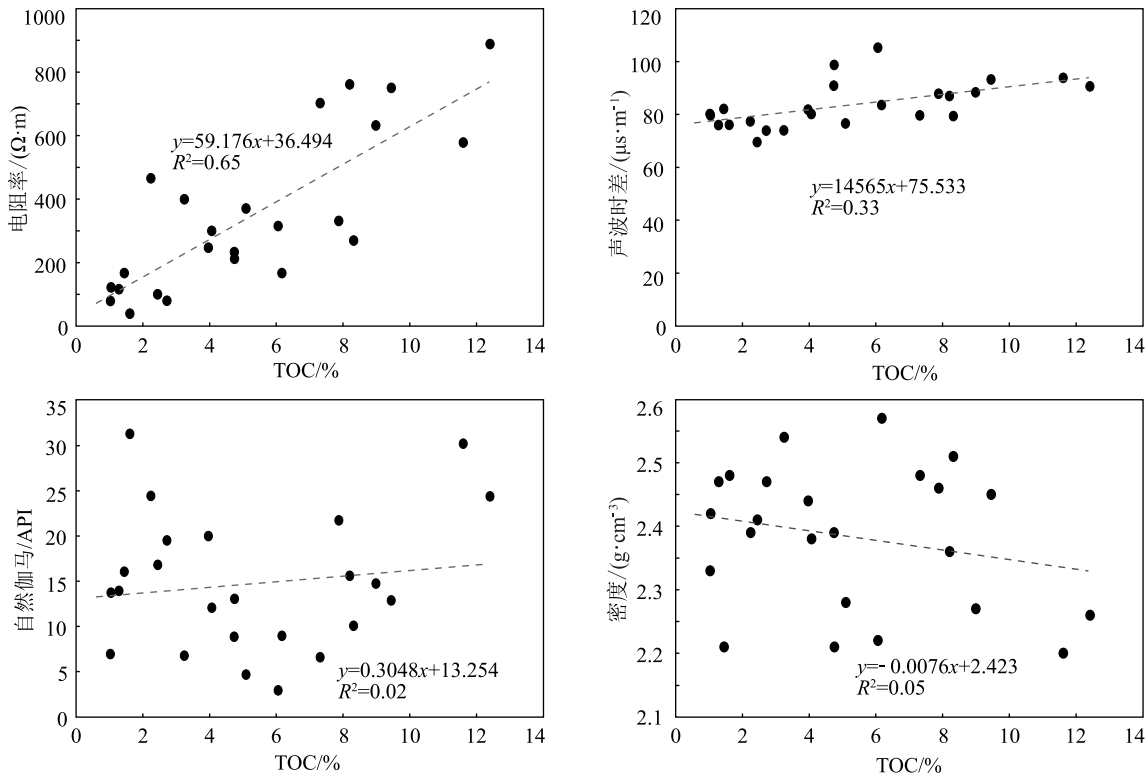
图 7 TOC 与电阻率、密度、声波时差、自然伽马相关性
