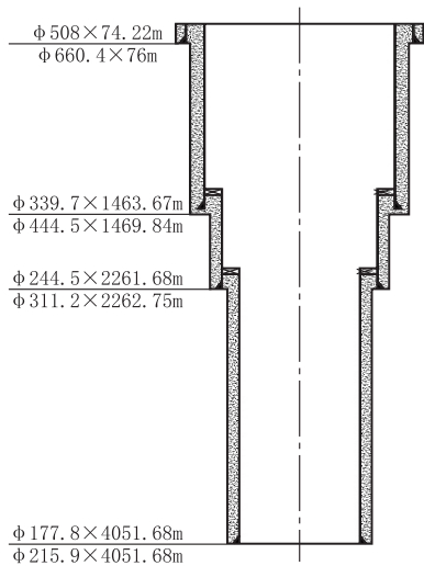
图 1 CGSD-01 井井身结构
