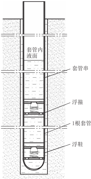
图 2 一开浮力下管示意图
