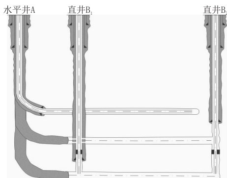
图3 多分支井技术在天然碱多层共采中的应用
