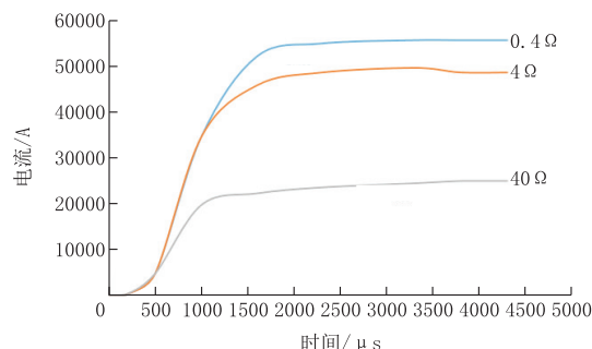
图 3 回路电阻对脉冲电流的影响
