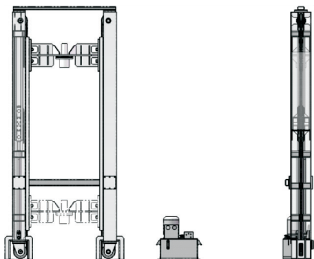
图2 液动锤固定台架结构示意图
