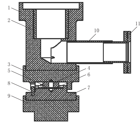
1—铁砧; 2—适应套; 3—上盖板; 4—上垫片; 5—传感器; 6—下垫片; 7—下盖板; 8—定位销; 9—基座; 10—出水管; 11—背压阀
