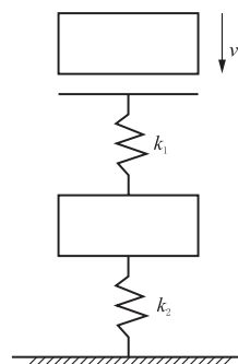
图3 冲击模型
