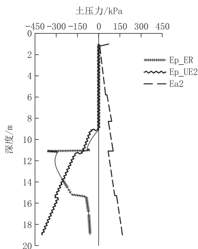
图 4 C'D'处基坑土压力
