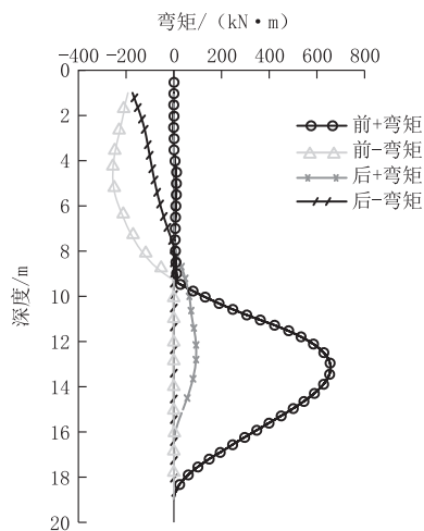
图 5 前后排桩弯矩
