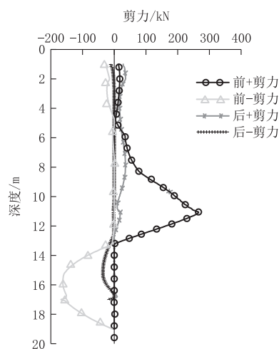
图 6 前后排桩剪力
