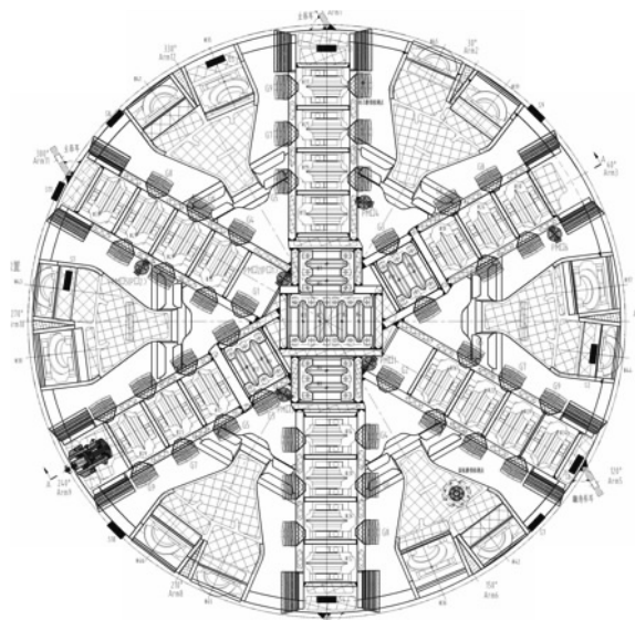
图 2 487 号盾构机刀盘结构
