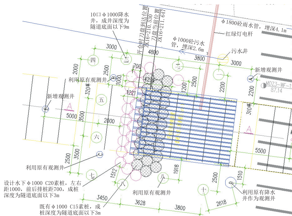
图6 第二次开仓换刀加固图
