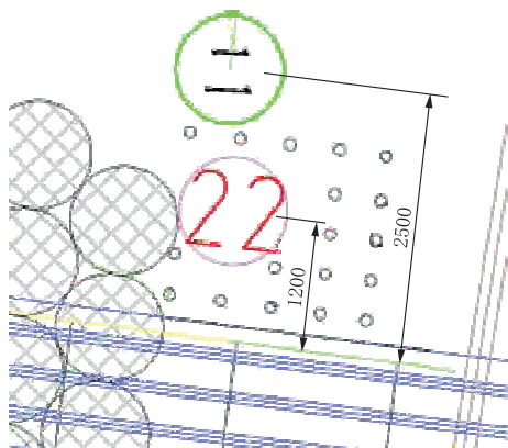
图7 22号桩周边钻孔注浆加固示意
