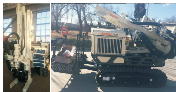
图 3 Geoprobe 7822DT 型钻机
