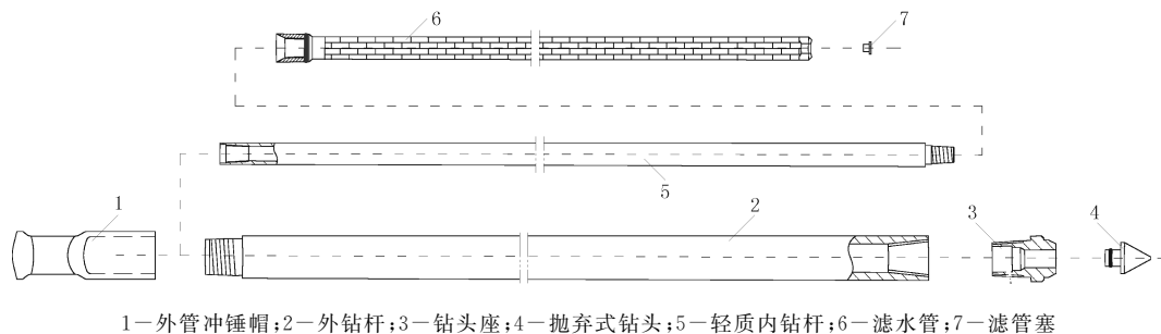
图 8 临时取水钻具组合示意图
