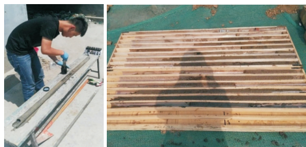
图 7 采取原状土样
