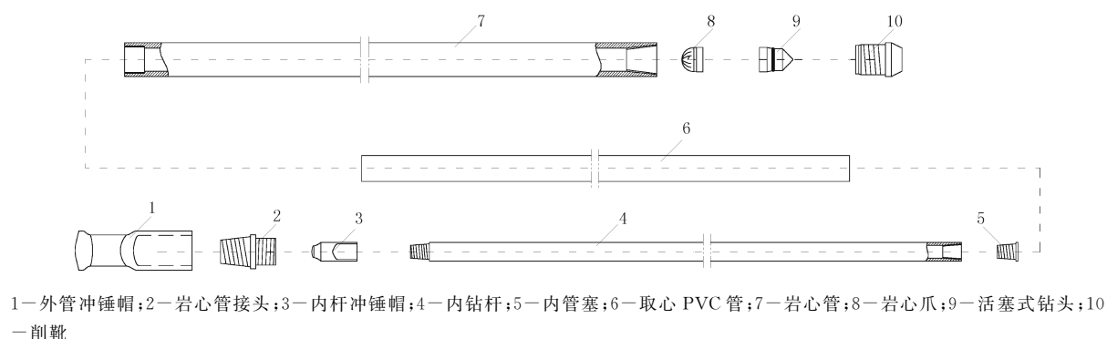
图 5 提钻取心钻具组合示意图
