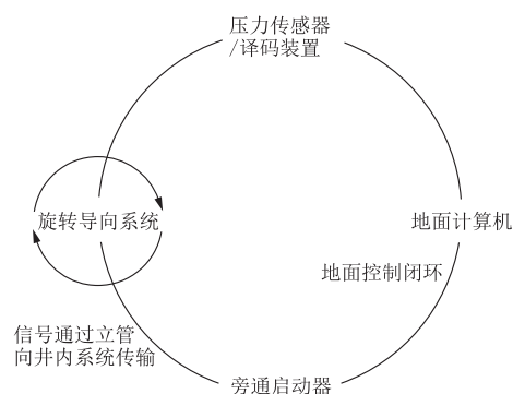
图 1 旋转导向闭环系统
