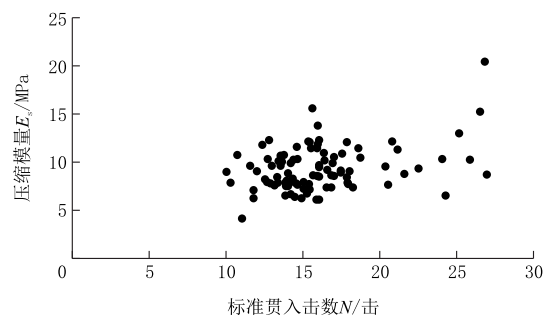
图2 标准贯入击数 N 与压缩模量 E_s 散点图
