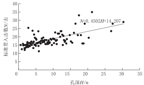
图1 标准贯入击数 N 与孔深 H 散点图
