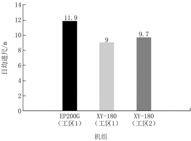
图 2 不同钻机的施工效率对比
