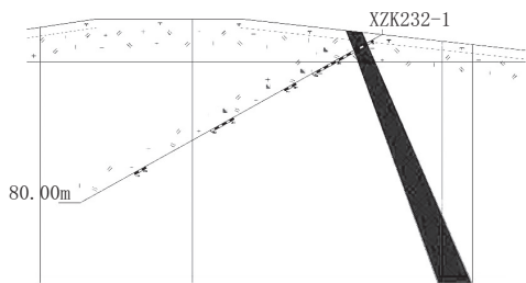
图 2 小倾角钻孔实际示意图
