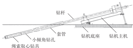
图 3 小倾角钻孔施工结构示意图
