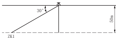
图 1 小倾角钻孔布设示意图
