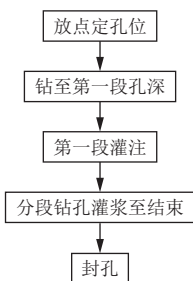
图4 深层固结单孔施工工艺流程
