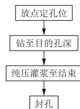
图 3 表层封堵单孔施工工艺流程
