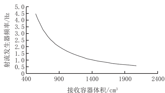
图8 射流发生器出口冲击频率与接收容器容积的关系曲线
