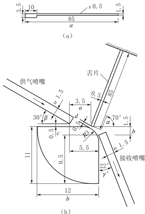
图9 方位角传感器中舌片(a)和射流发生器(b)尺寸、角度
