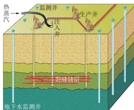
图8 雪佛龙 CRUSH 技术原理示意 [17,27-28]
