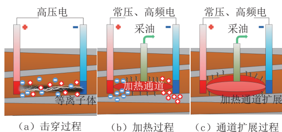
图7 吉林大学高压-工频电加热(HVF)技术原理示意 [23]
