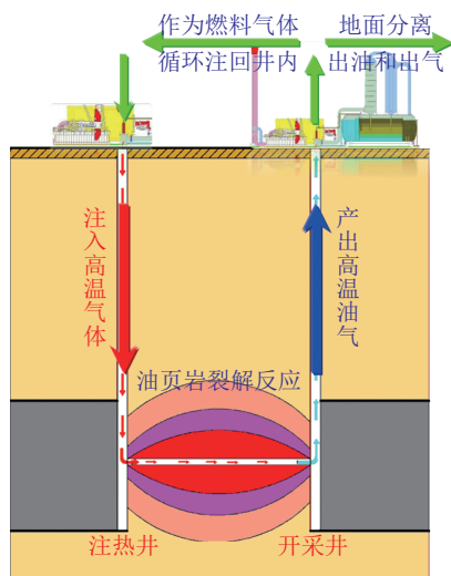
图3 吉林大学TSA技术原理示意
