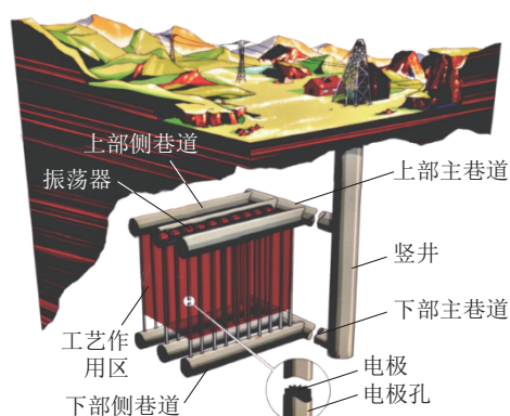
图13 LINL 射频技术原理示意图 [35]
