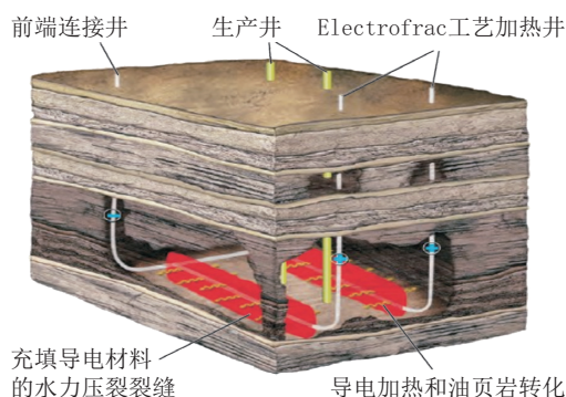
图6 埃克森美孚公司的 Electrofrac™ 技术原理示意图 [17,24]
