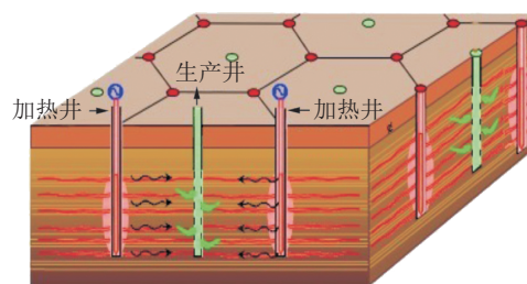
图5 壳牌ICP技术原理示意 [17,24]
