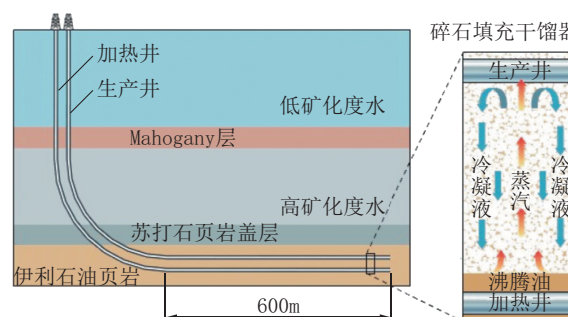
图9 美国页岩油公司 CCR 技术原理示意 [17,30]
