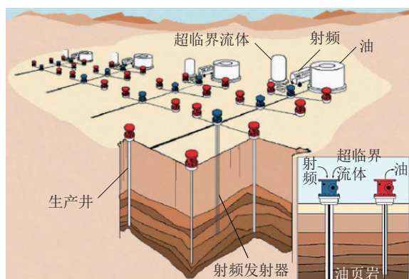
图12 Raytheon公司 RF/CF 技术原理示意图 [34]
