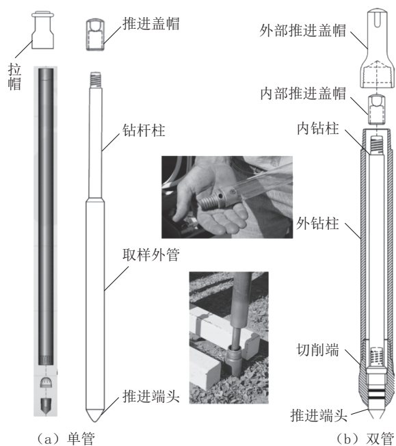
图5 单管(a)和双管(b)组合结构
