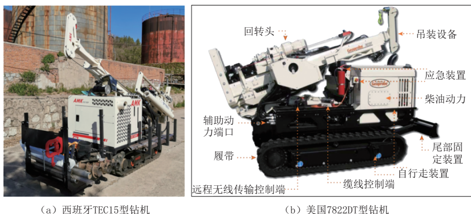
图3 直推钻机结构
