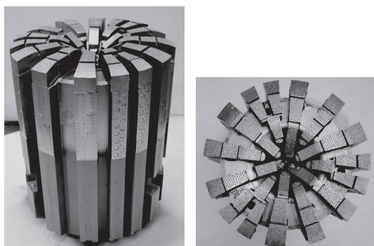
图2 Ø333 mm 表孕镶金刚石全面钻头
