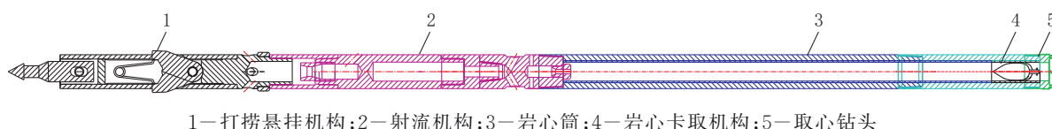
图3 海洋砂质地层绳索取心钻具
