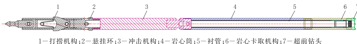
图4 液动冲击绳索取心钻具
