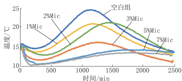
图5 水泥浆水化放热温度-时间曲线
