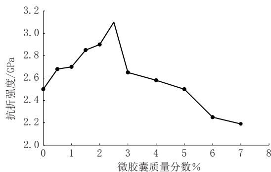
图7 水泥试件抗折强度
