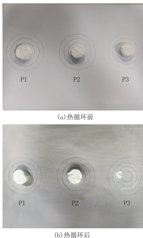
图2 热循环前与热循环后样品泄露情况
