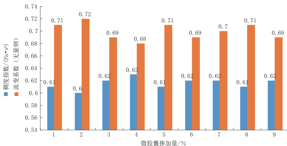
图4 相变微胶囊对水泥浆流变性能的影响
