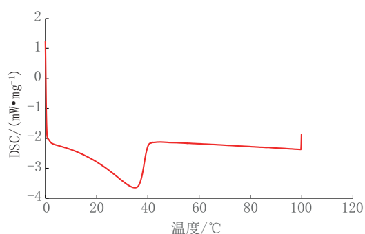
图3 相变微胶囊的DSC曲线
