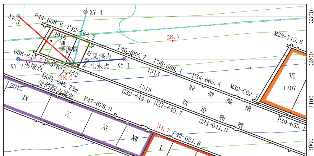
图1 工作面示意
