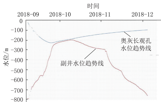
图4 副井排水过程中奥灰长观孔和副井水位变化趋势 (2018年9月10日—12月18日)
