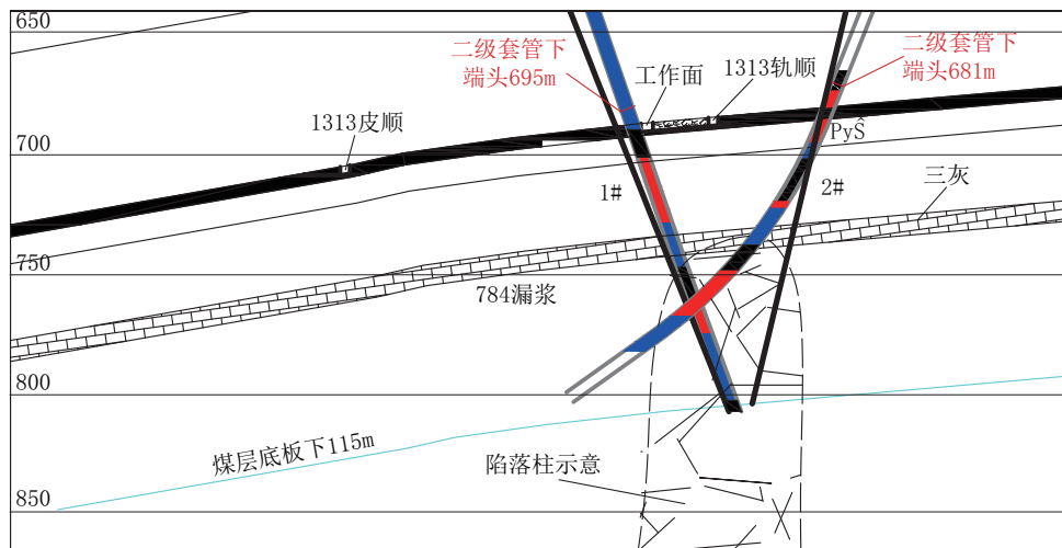
图3 陷落柱示意
