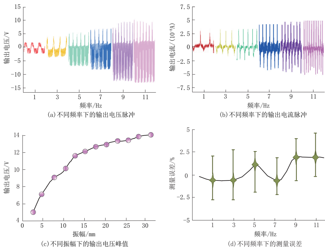
图2 自供电振动传感器测量特征
