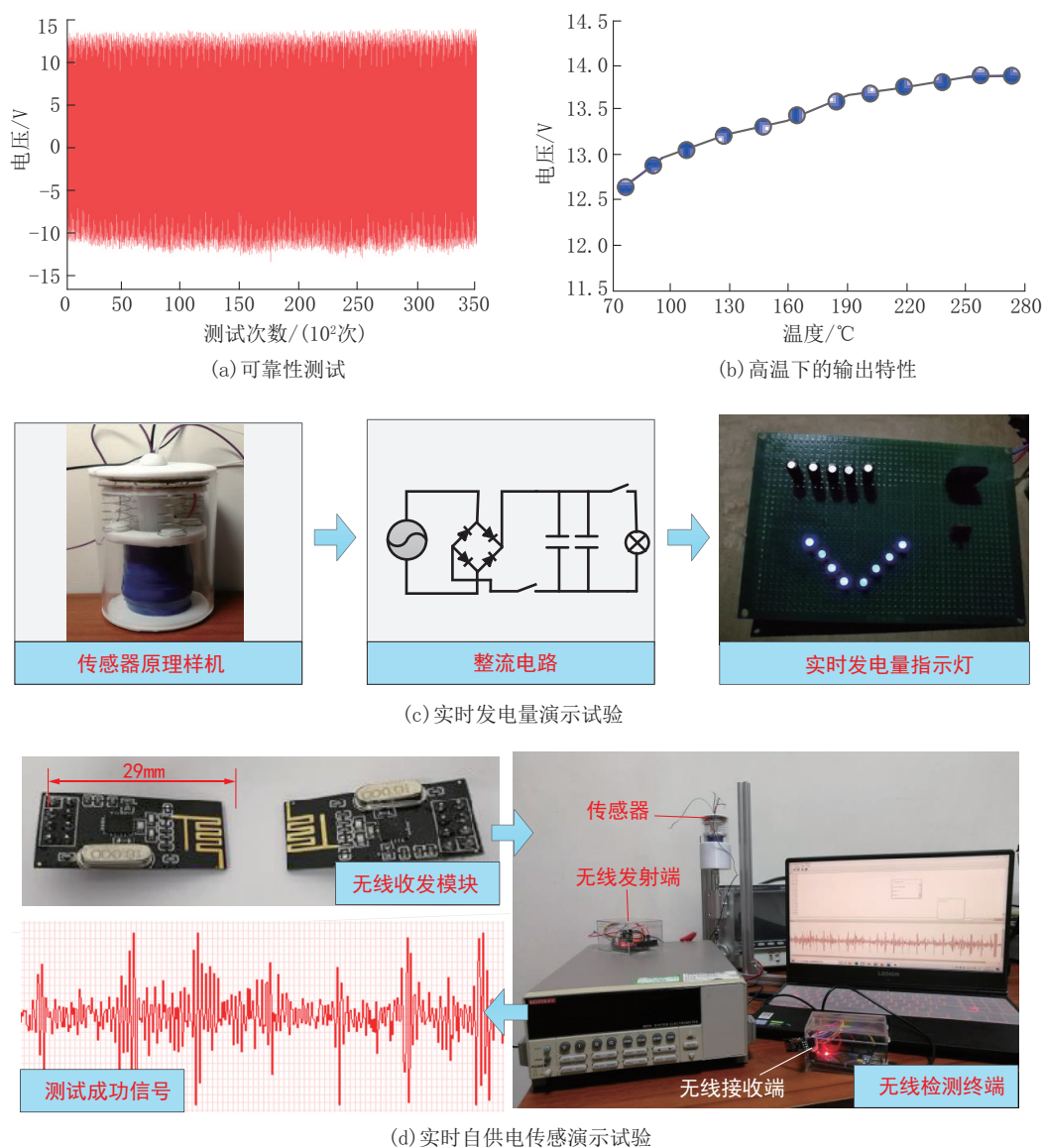
图4 自供电振动传感器应用试验
