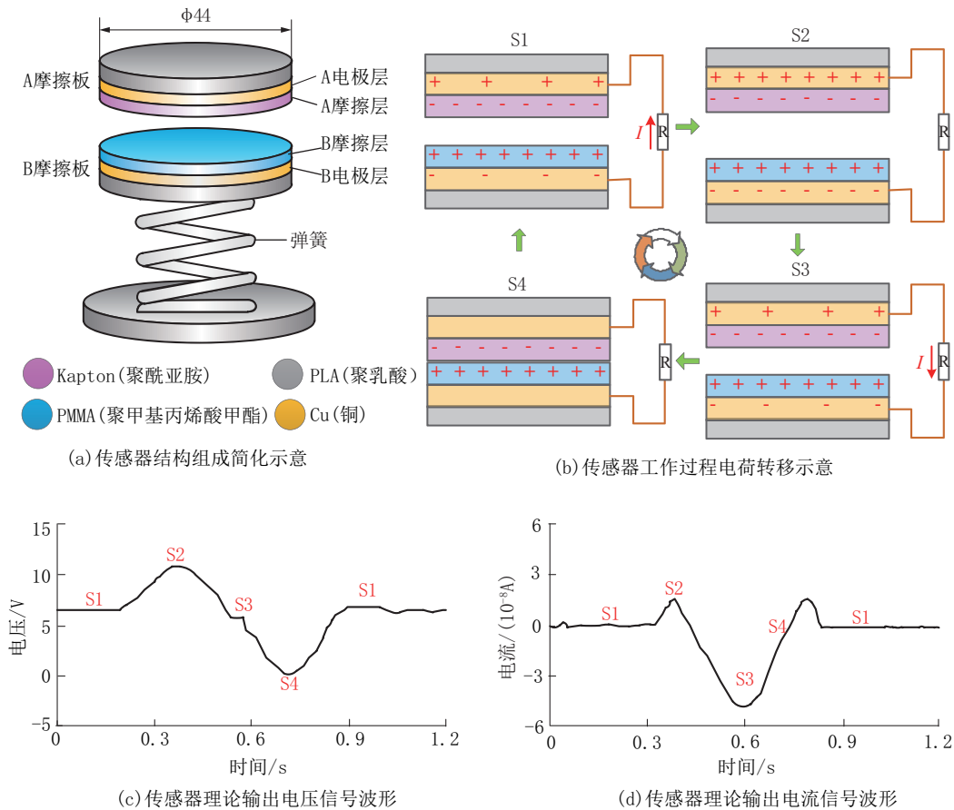
图1 自供电振动传感器工作原理示意
