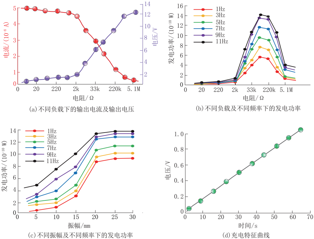
图3 自供电振动传感器发电特征
