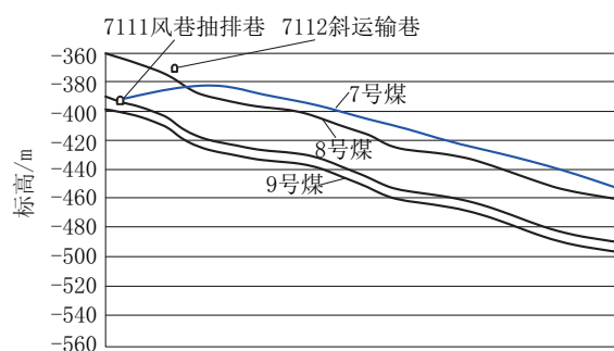
图11 钻孔轨迹剖面示意
