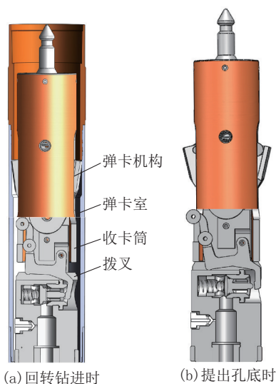
图4 内管总成上端部保压密封动作示意
