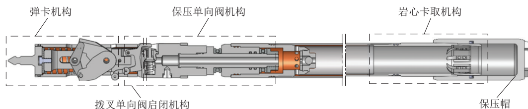
图3 \varnothing 75 mm 保压绳索取心钻具内管总成
