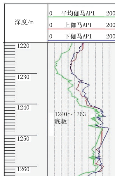
图4 轨迹下切后返回煤层
