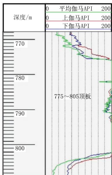
图3 轨迹上切后返回煤层
