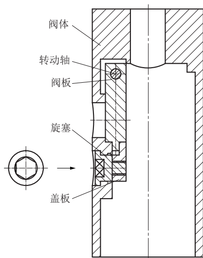
图2 连续循环接头(CCJ)示意
