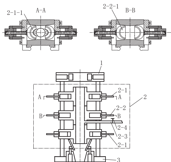
1—背钳;2—自动钻井液切换系统;2-1—半封闸板防喷器;2-1-1—半圆环形闸板;2-2—全封闸板防喷器;2-2-1—半圆形闸板;2-3—钻井液旁通管路;2-4—开关阀门;3—传扭动力卡瓦
