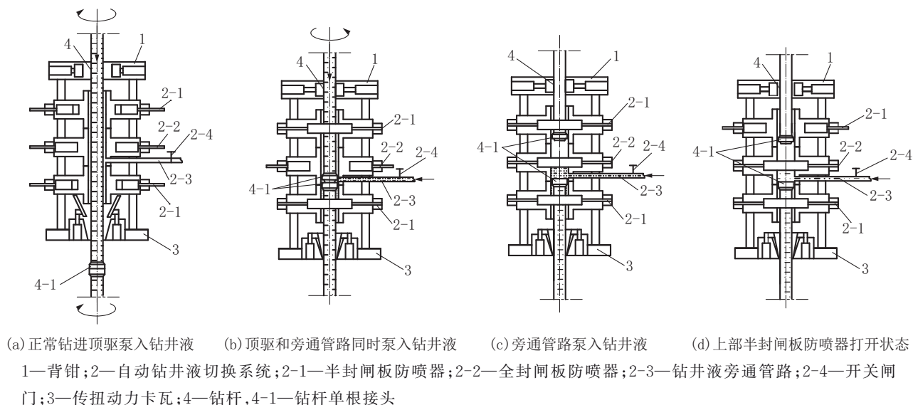
图4 拆卸钻杆时钻井液连续循环工作原理
