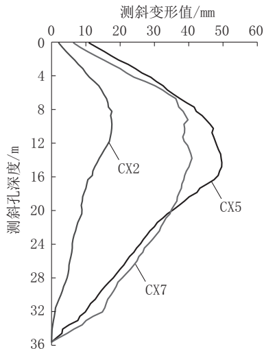
图7 地连墙测斜变形监测数据
