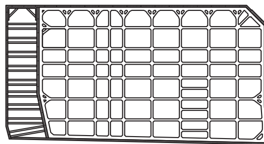
图4 第二、三道支撑平面布置
