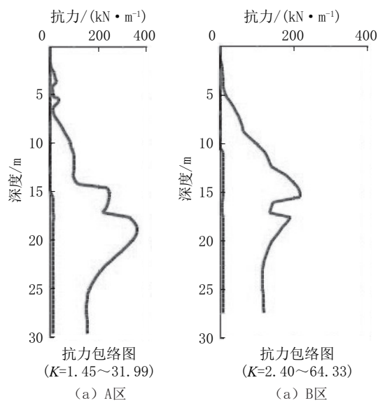
图5 基坑围护剖面计算结果
