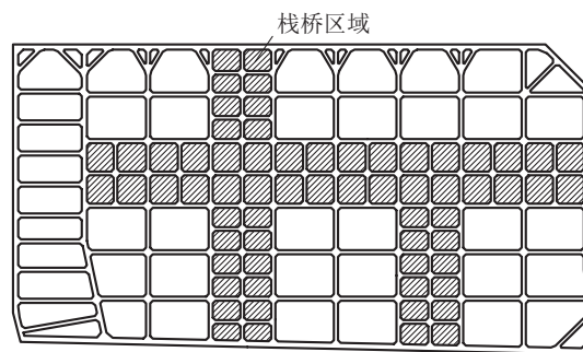
图3 第一道支撑平面布置
