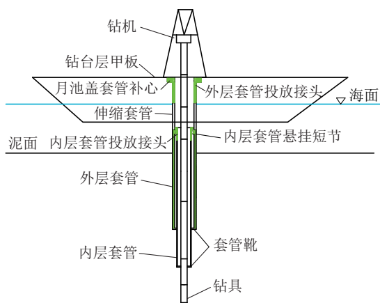
图2 下入两层套管的伸缩套管工艺方法示意
