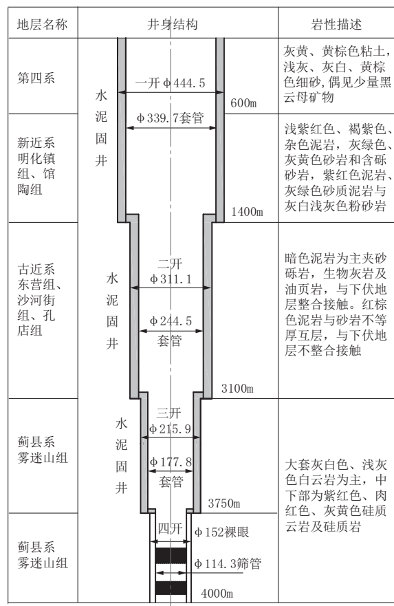
图2 JZ04井备用井身结构
