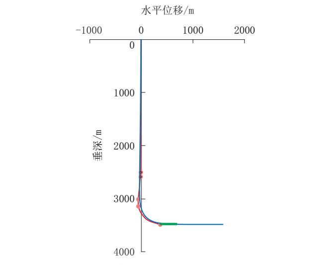
图6 苏14-19-34H1井垂直投影 Fig.6 Vertical projection of Su 14-19-34H1
