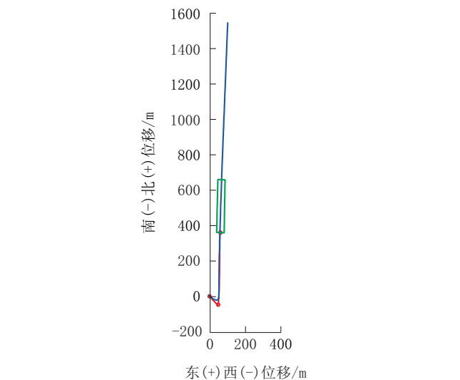
图5 苏14-19-34H1井水平投影 Fig.5 Horizontal projection of Su 14-19-34H1
