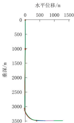
图8 苏14-19-34H2井垂直投影
