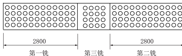
图5 单铣密排孔
