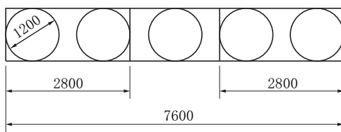
图8 引孔布置
