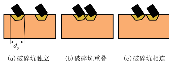
图4 冲击碎岩示意
