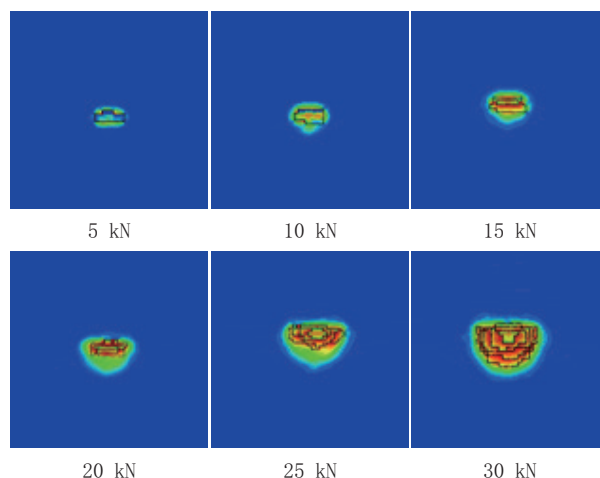
图6 横向破坏波及面积局部放大图
