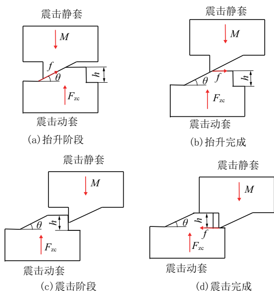
图3 震击机构不同状态下简化受力
