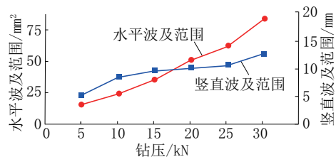
图7 不同钻压震击碎岩的影响
