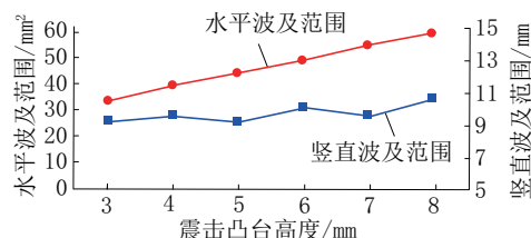
图8 不同震击凸台高度对碎岩的影响
