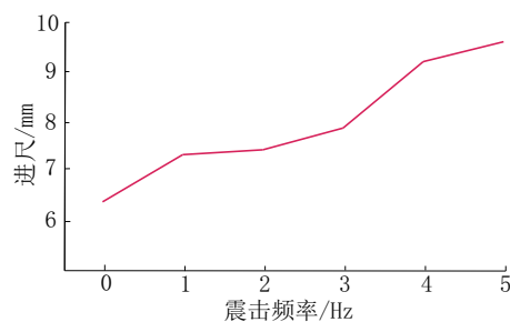
图9 不同频率碎岩的影响
