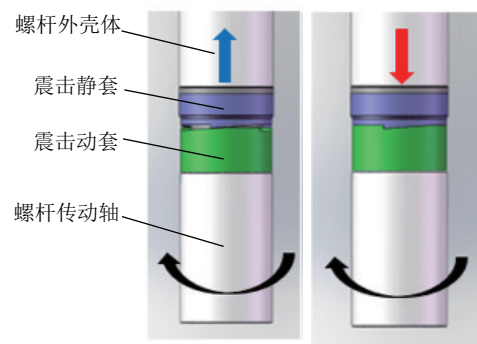
图2 震击机构结构及原理
