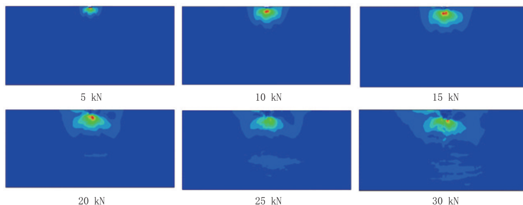
图5 震击破碎岩石的纵向波及范围结果
