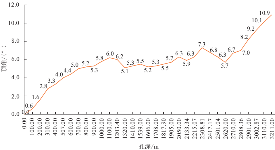
图 4 孔斜曲线 Fig.4 Inclinometer curve
