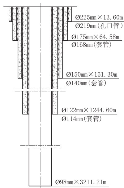
图2 钻孔结构
