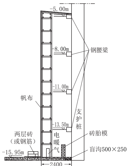
图5 2号区域侧壁渗漏部位防护措施
