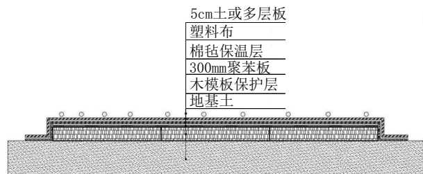
图4 覆土及西侧未开挖至基底区域保温断面图
