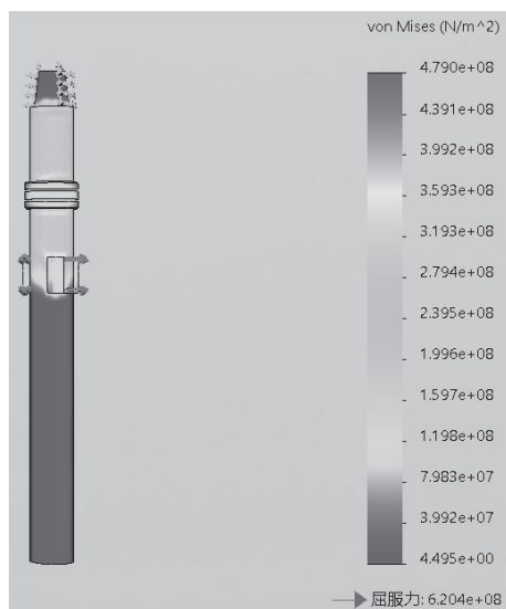
图3 传扭轴应力云图
