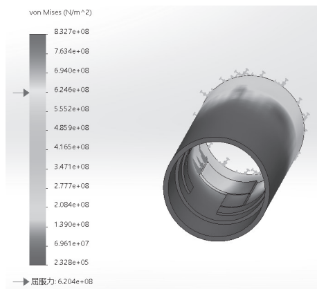
图4 传扭壳体塑性变形云图
