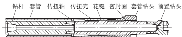
图1 跟管钻进原理示意
