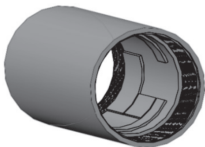
图5 传扭壳体
